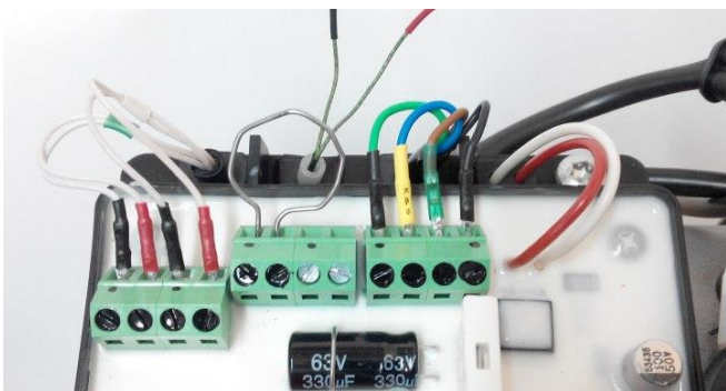
Рис. 6 – Перемычка
