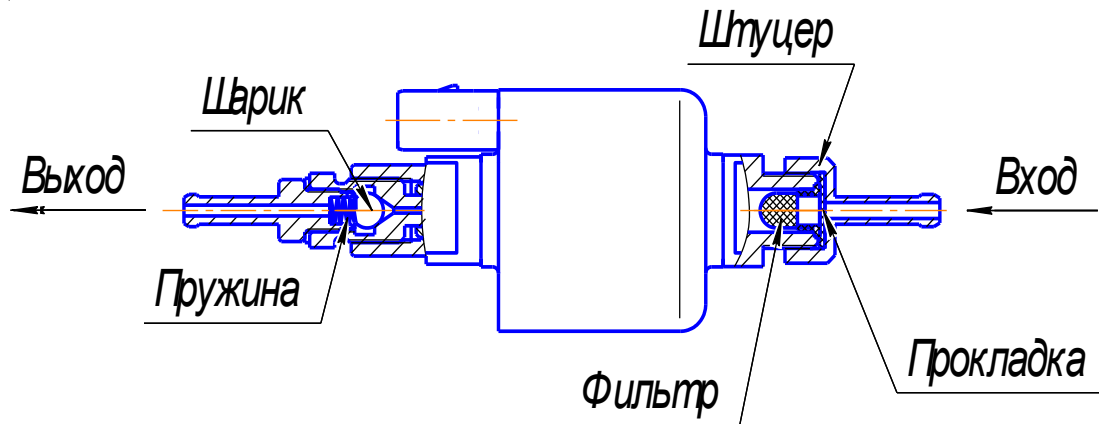
Рис. 14 - Топливный насос
