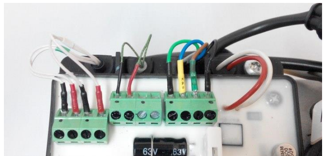
Рис. ба – Подключение ИП к БУ
