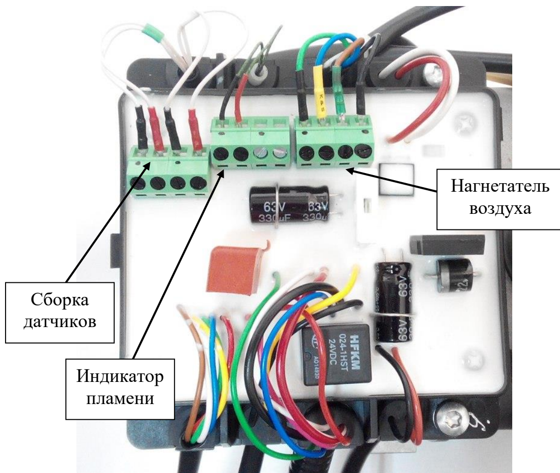
Рис.12 – Блок управления.
